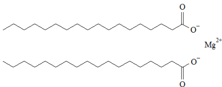
Рисунок 1. – Структурная формула магния стеарата
