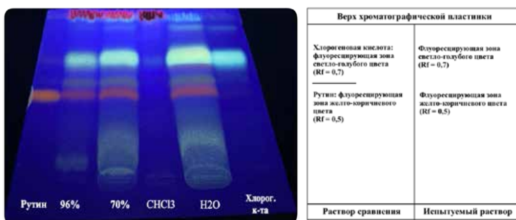
Рисунок 10. – ТСХ-хроматограмма извлечений из листьев борщевика Сосновского в системе муравьиная кислота : метилэтилкетон : вода : этилацетат (10 : 30 : 10 : 50)
