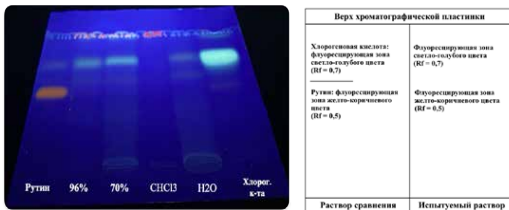
Рисунок 9. – ТСХ-хроматограмма извлечений из стеблей борщевика Сосновского в системе муравьиная кислота : метилэтилкетон : вода : этилацетат (10 : 30 : 10 : 50)
