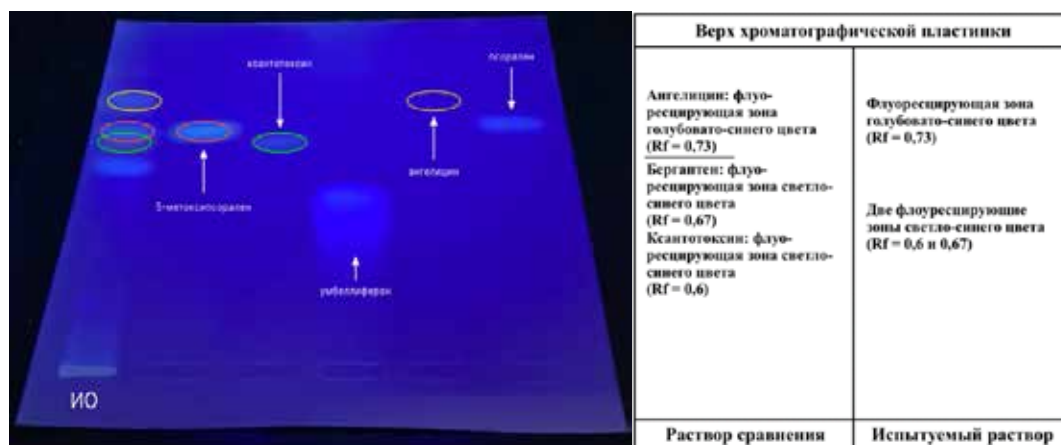
Рисунок 2. – ТСХ-хроматограмма хлороформного извлечения из корней борщевика Сосновского в системе петролейный эфир : этилацетат : бензол (2 : 1 : 0,5)
