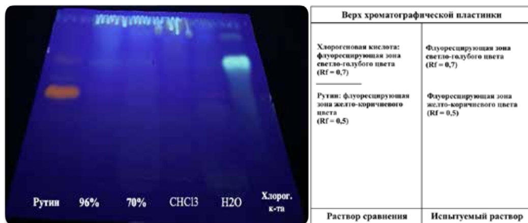
Рисунок 11. – ТСХ-хроматограмма извлечений из семян борщевика Сосновского в системе муравьиная кислота : метилэтилкетон : вода : этилацетат (10 : 30 : 10 : 50)
