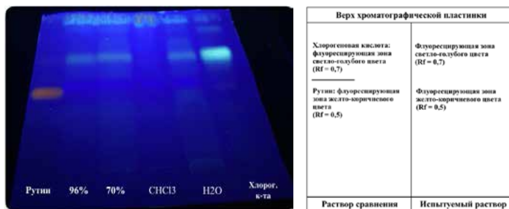
Рисунок 7. – ТСХ-хроматограмма извлечений из корней борщевика Сосновского в системе муравьиная кислота : метилэтилкетон : вода : этилацетат (10 : 30 : 10 : 50)
