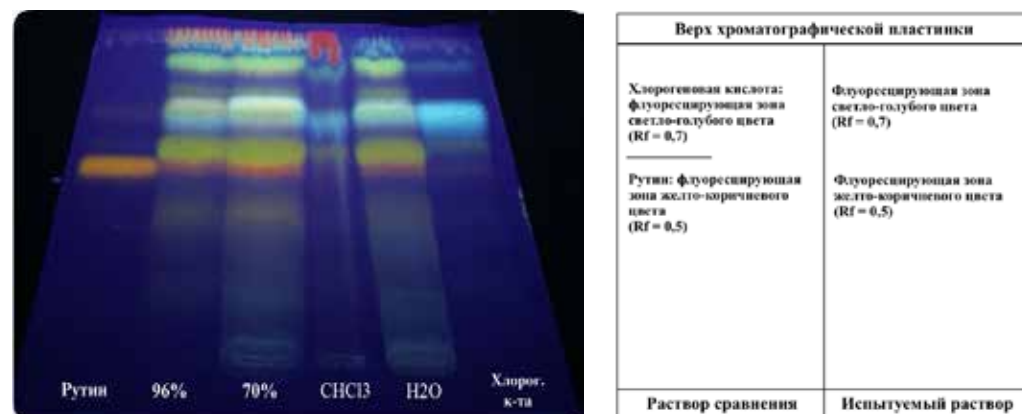
Рисунок 8. – ТСХ-хроматограмма извлечений из соцветий борщевика Сосновского в системе муравьиная кислота : метилэтилкетон : вода : этилацетат (10 : 30 : 10 : 50)
