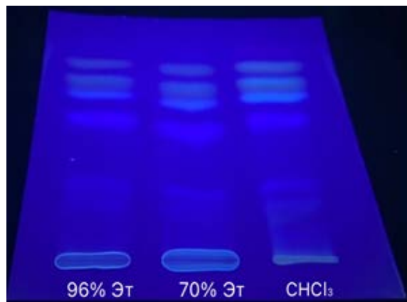
Рисунок 1. – ТСХ-хроматограмма извлечений из корней борщевика Сосновского в системе петролейный эфир : этилацетат : бензол (2 : 1 : 0,5)
