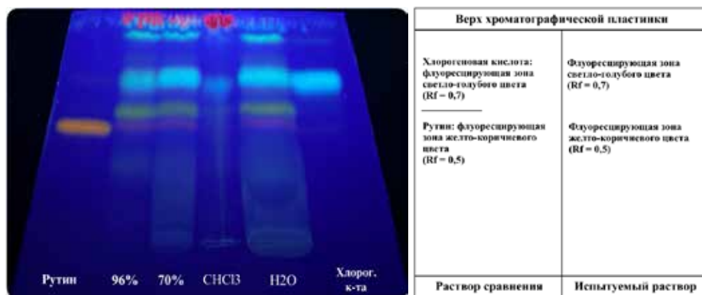
Рисунок 6. – ТСХ-хроматограмма извлечений из травы борщевика Сосновского в системе муравьиная кислота : метилэтилкетон : вода : этилацетат (10 : 30 : 10 : 50)
