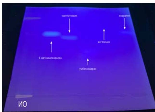
Рисунок 5. – ТСХ-хроматограмма хлороформного извлечения из травы борщевика сибирского в системе петролейный эфир : этилацетат : бензол (2 : 1 : 0,5)
