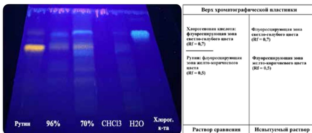
Рисунок 13. – ТСХ-хроматограмма извлечений из стеблей борщевика сибирского в системе муравьиная кислота : метилэтилкетон : вода : этилацетат (10 : 30 : 10 : 50)
