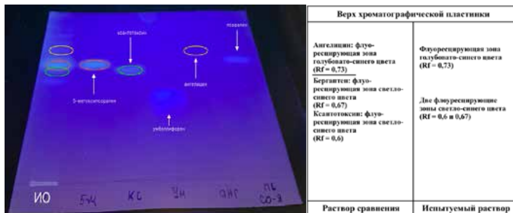
Рисунок 3. – ТСХ-хроматограмма хлороформного извлечения из соцветий борщевика Сосновского в системе петролейный эфир : этилацетат : бензол (2 : 1 : 0,5)
