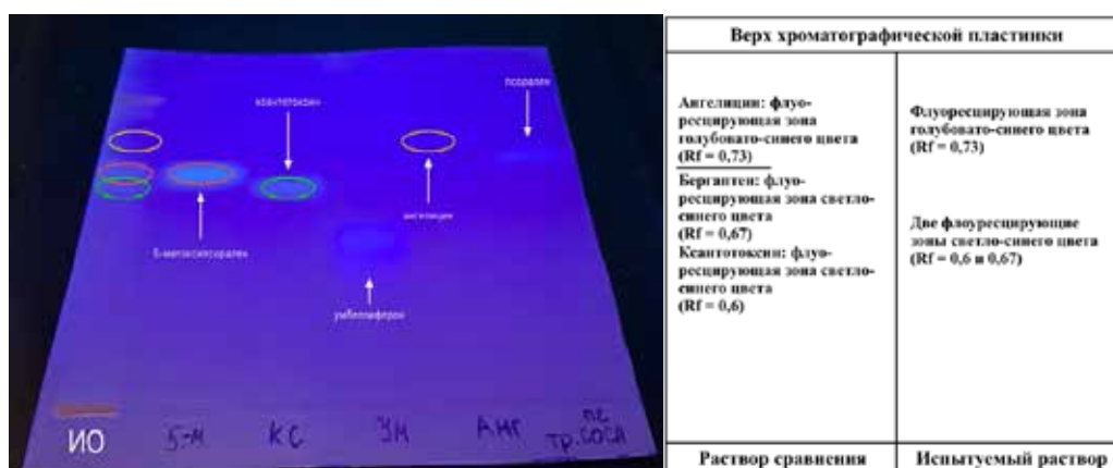
Рисунок 4. – ТСХ-хроматограмма хлороформного извлечения из травы борщевика Сосновского в системе петролейный эфир : этилацетат : бензол (2 : 1 : 0,5)
